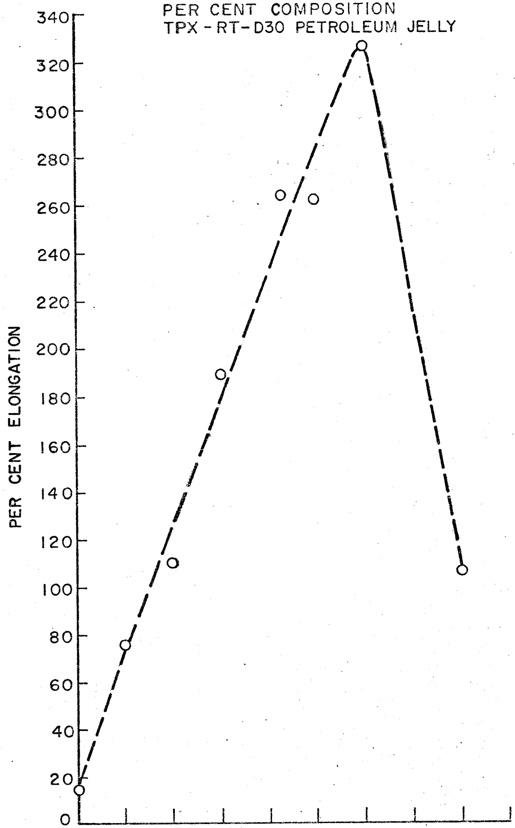
% TPX-RT-D30 : 100 95 90 85 80 75 70 65 60 55 % PETROLEUM JELLY : 0 5 10 15 20 25 30 35 40 45 GRAPH 3
